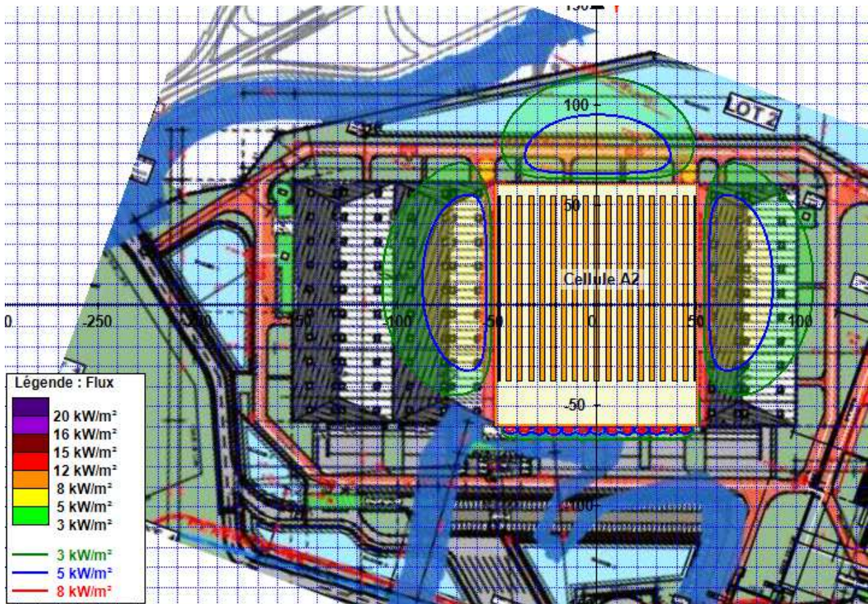
Figure 2 – Cartographie des flux thermiques – cellule A2 (palette type 2662) – Bâtiment A
