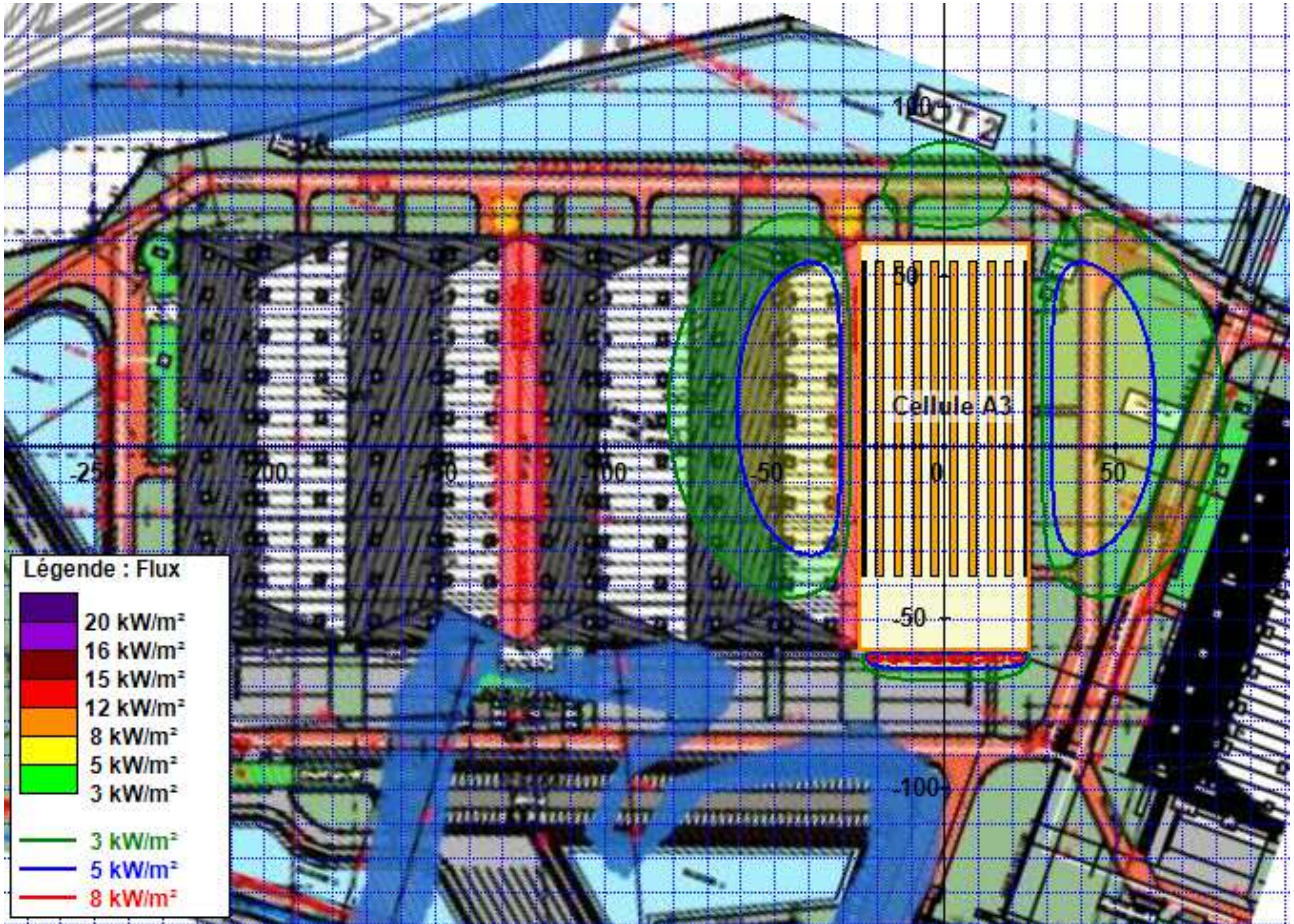
Figure 3 – Cartographie des flux thermiques – cellule A3 (palette type 2662) – Bâtiment A
