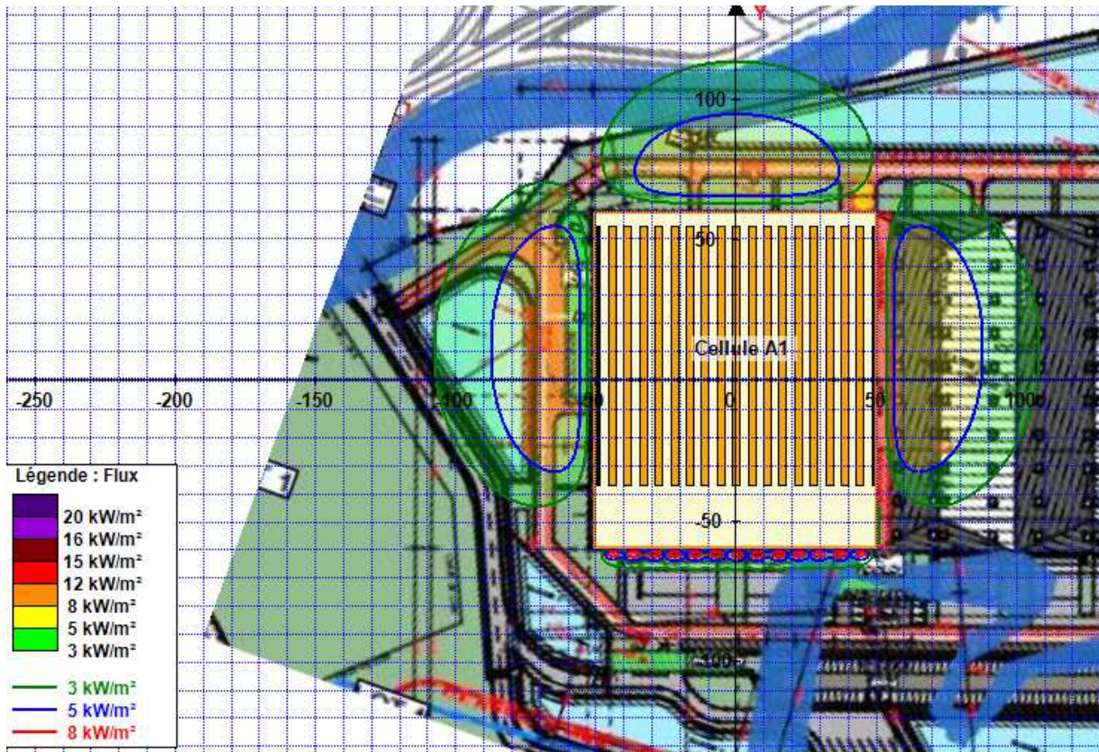
Figure 1 – Cartographie des flux thermiques – cellule A1 (palette type 2662) – Bâtiment A
